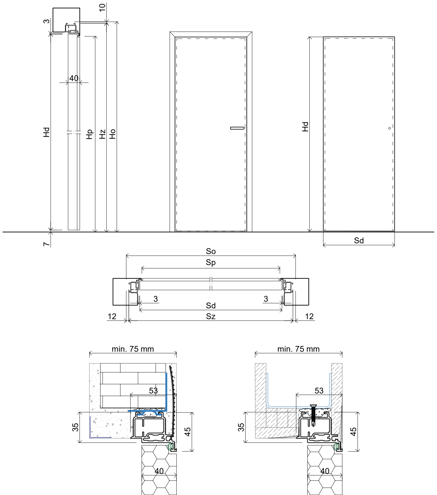
Wymiary standardowe dla drzwi otwieranych do wewnątrz
