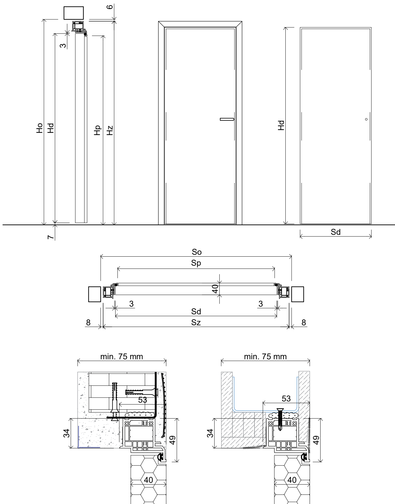
Wymiary standardowe dla drzwi otwieranych do wewnątrz
